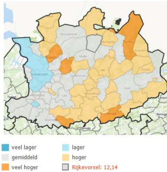
Figuur 14 | Energieverbruik door fossiele brandstoffen in MWh per huishouden (2017)
