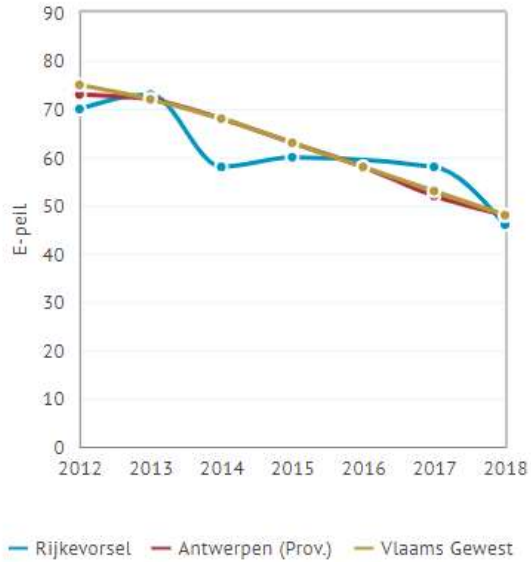
Figuur 6 | Evolutie gemiddeld E-peil voor nieuwbouwwoningen (2012-2018)
