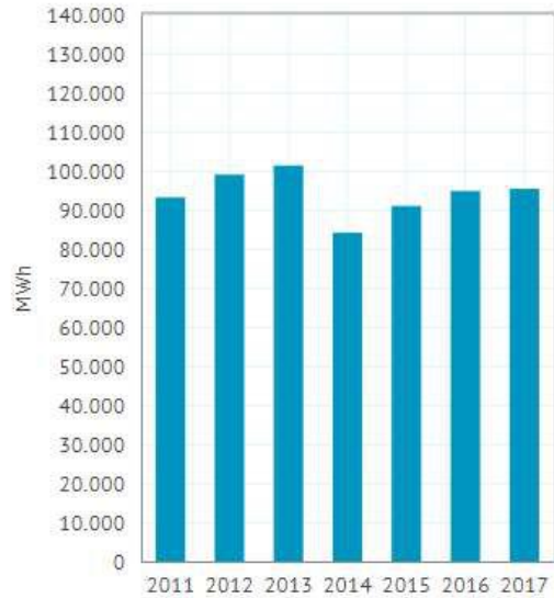
Figuur 9 | Evolutie totaal energieverbruik door huishoudens in Rijkvorsel (2011-2017)
