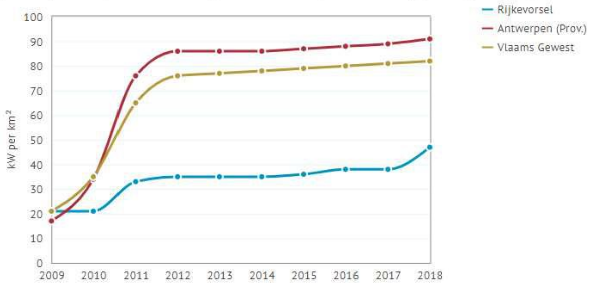
Figuur 51 | Evolutie geïnstalleerd vermogen PV-installaties groter dan 10 kW, per km 2 (2009-2018)
